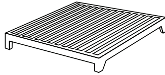
Lattes rigides avec espacement maximum de 4'' ou lattes flexibles avec espacement maximum de 2''
